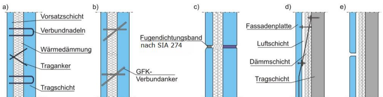
Bild 2: Prinzipielle Fassadenausbildungen und typische Fugendetails, a) b) und c) Sandwichelemente, d) und e) vorgehängte Fassadenplatten
