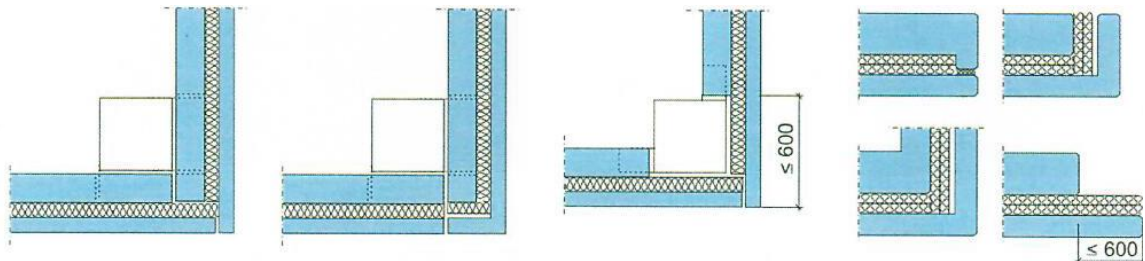
Bild 3: Ecklösungen mit der Tragschicht zwischen und vor den Stützen und übliche Randausbildungen
